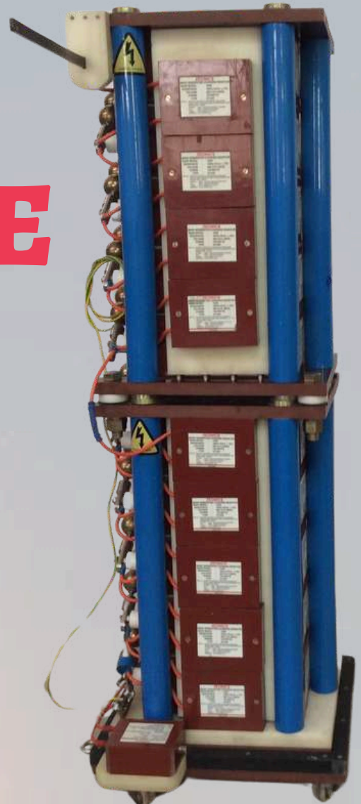
Million Volt Generator
